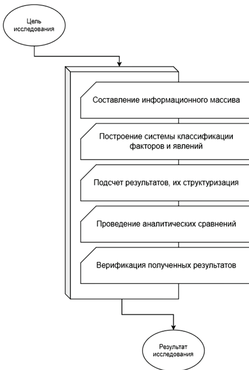
Рис. 1. Алгоритм ивент-анализа
